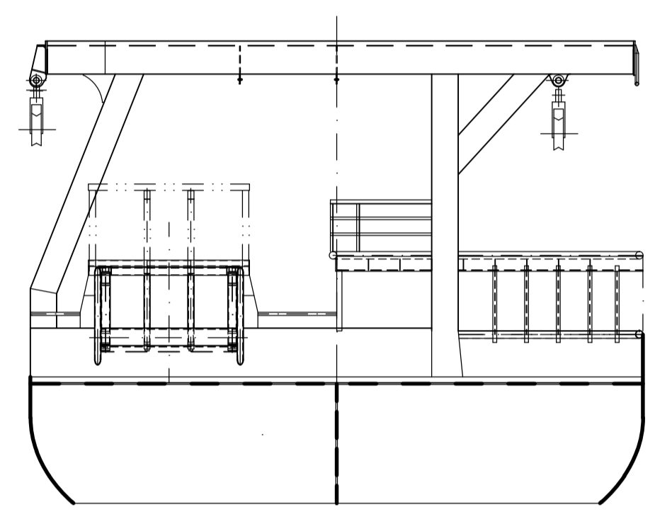
TRANSOM
